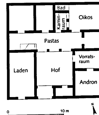
Olynthos, Pastas-Haus, 1. H. 4. Jh. v. Chr. (Grundriß).
